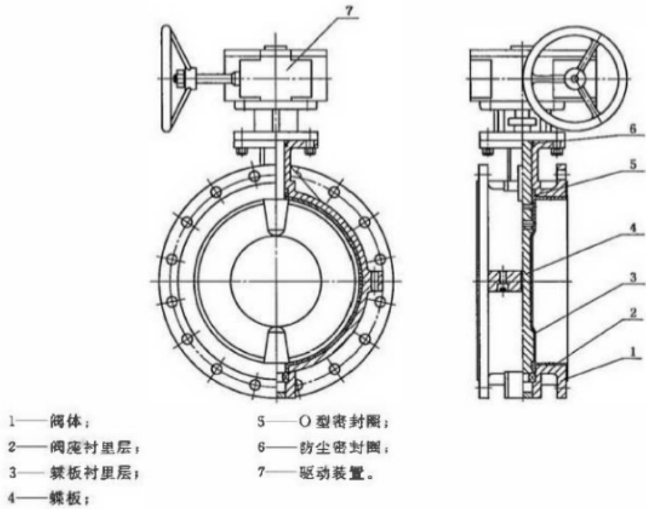
图 1 双法兰式连接蝶阀
