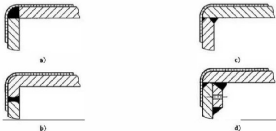
图 6 角焊缝
