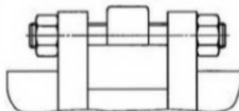
b) 无法兰
