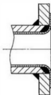
图 7 法兰焊缝
