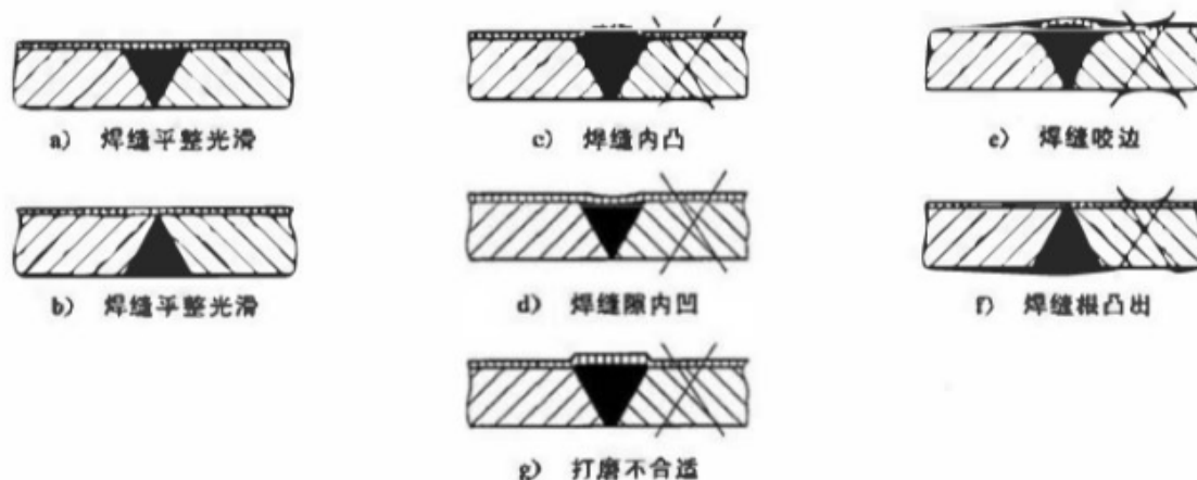
图 5 对接焊缝
